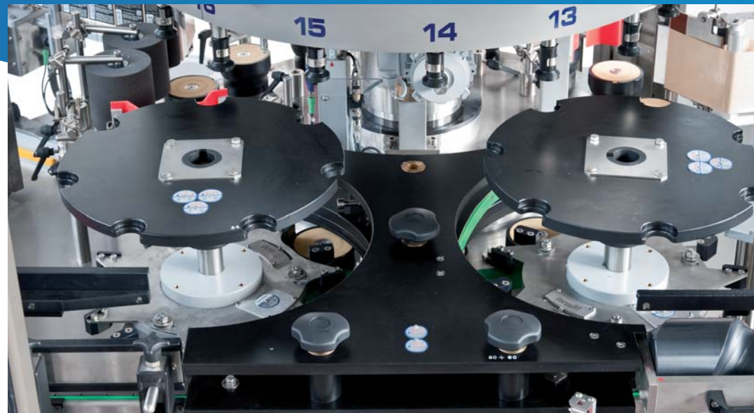
Stelle entrata/uscita multiformato Multi-format in/out star wheels Estrellas multiformato para entrada y salida
